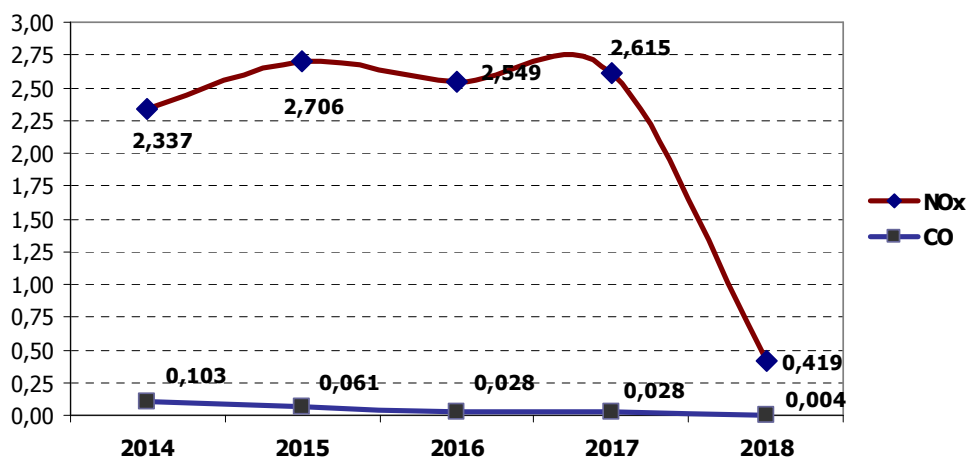
Vývoj produkce NO x a CO v období 2014-2018 (v t)
